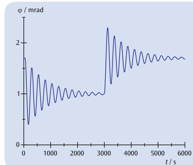
Рис. 2: Зависимость угла отклонения крутильного маятника от времени, когда положение измерения двух больших свинцовых шариков изменяется дважды
